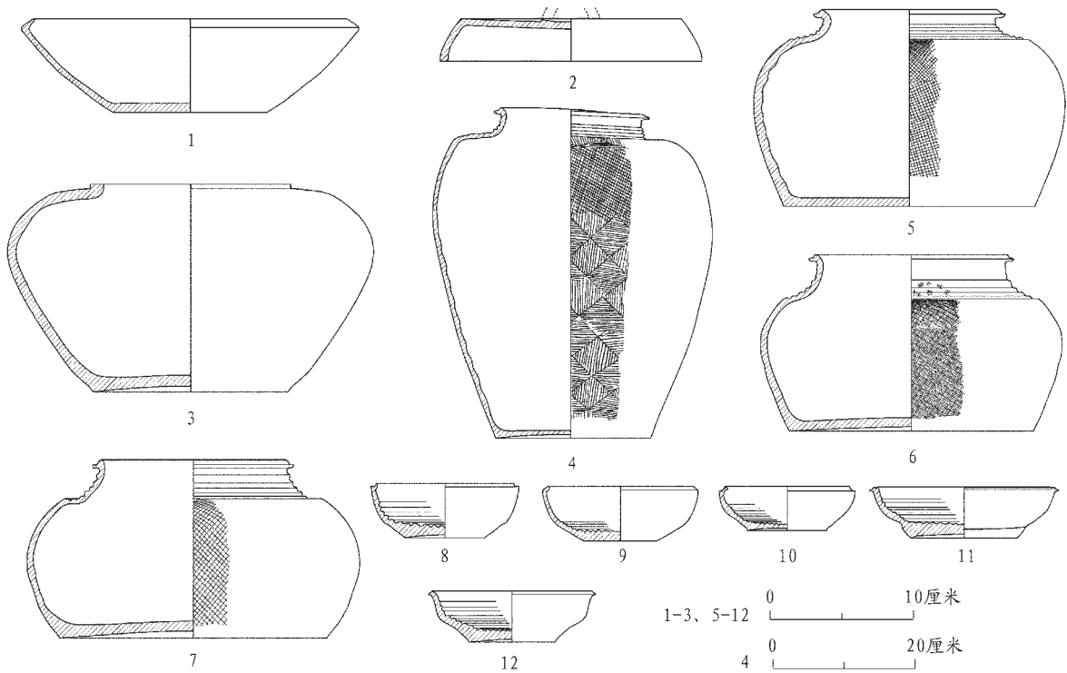
图八// M2出土器物
