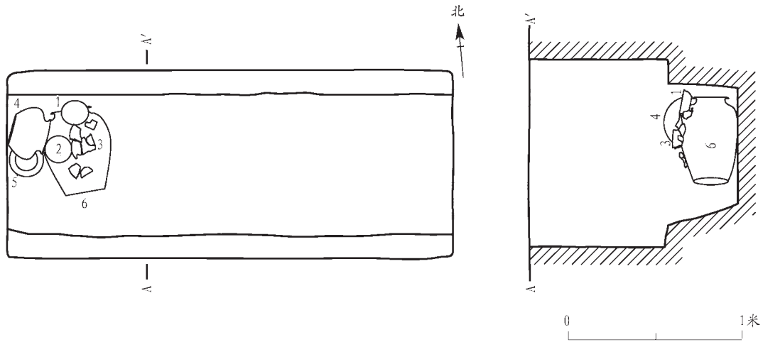
图九// M3平面图、剖视图
