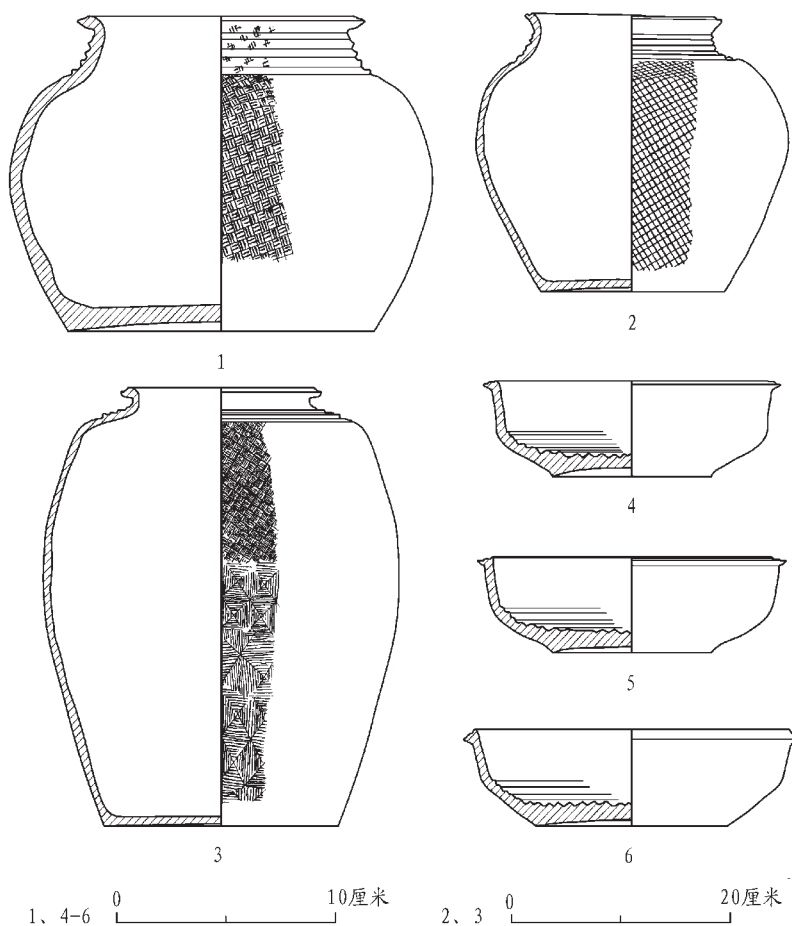
图十// M3出土器物
