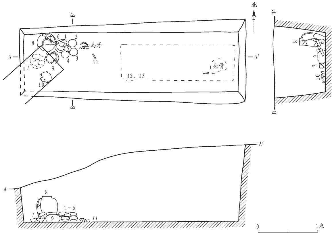
图四// M1平面图、剖视图
