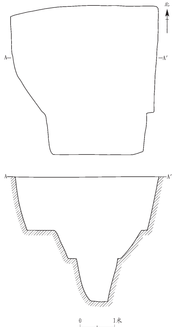
图十三// H2平、剖面图
